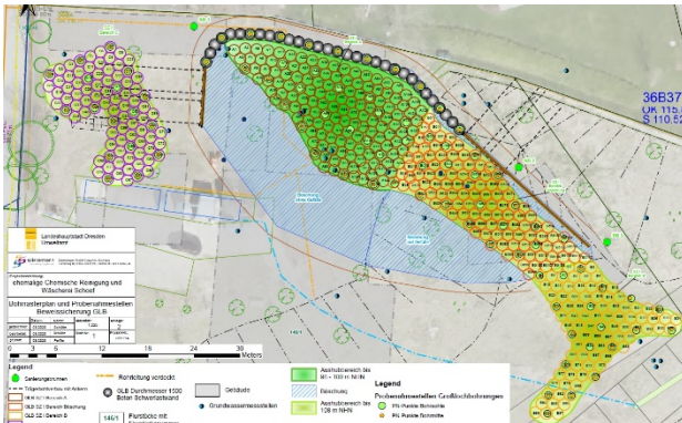
Bild 1: Bohrraster
