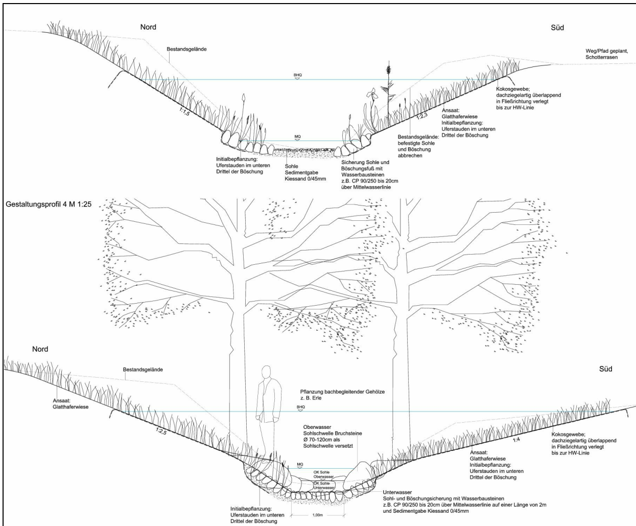
Abb. 7: Kaitzbach Altstrehlen 1. BA Querprofile, 16.01.2017
