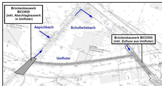
Abb. 4: Planung - schematischer Lageplan Brücken und Umfluter, 25.11.2014
