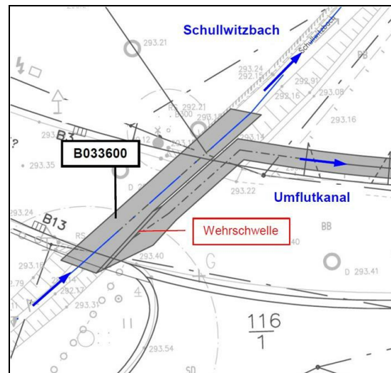
Abb. 5: Planung - Einlauf in Umfluter, 25.11.2014
