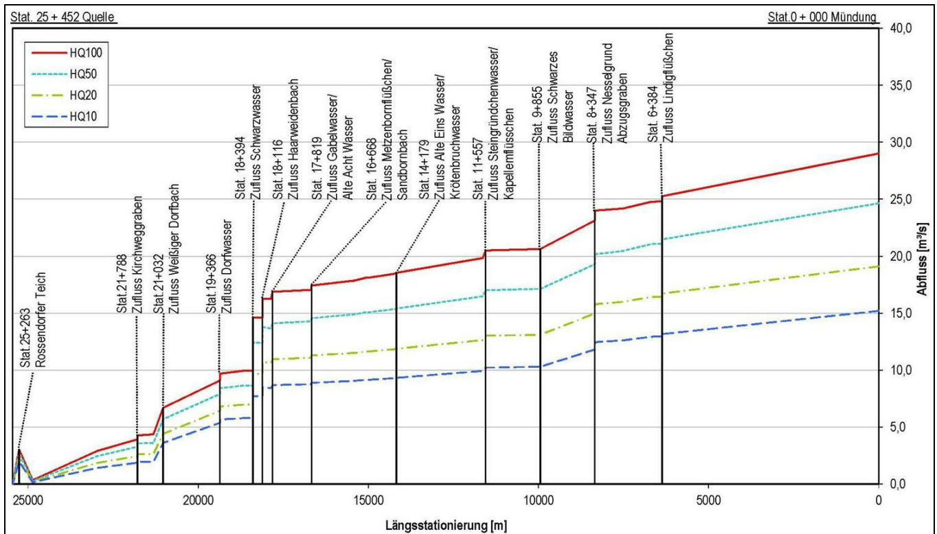
Abb. 43: Hochwasserabfluss in der Prießnitz - Hydrologischer Längsschnitt; 08.04.2019
