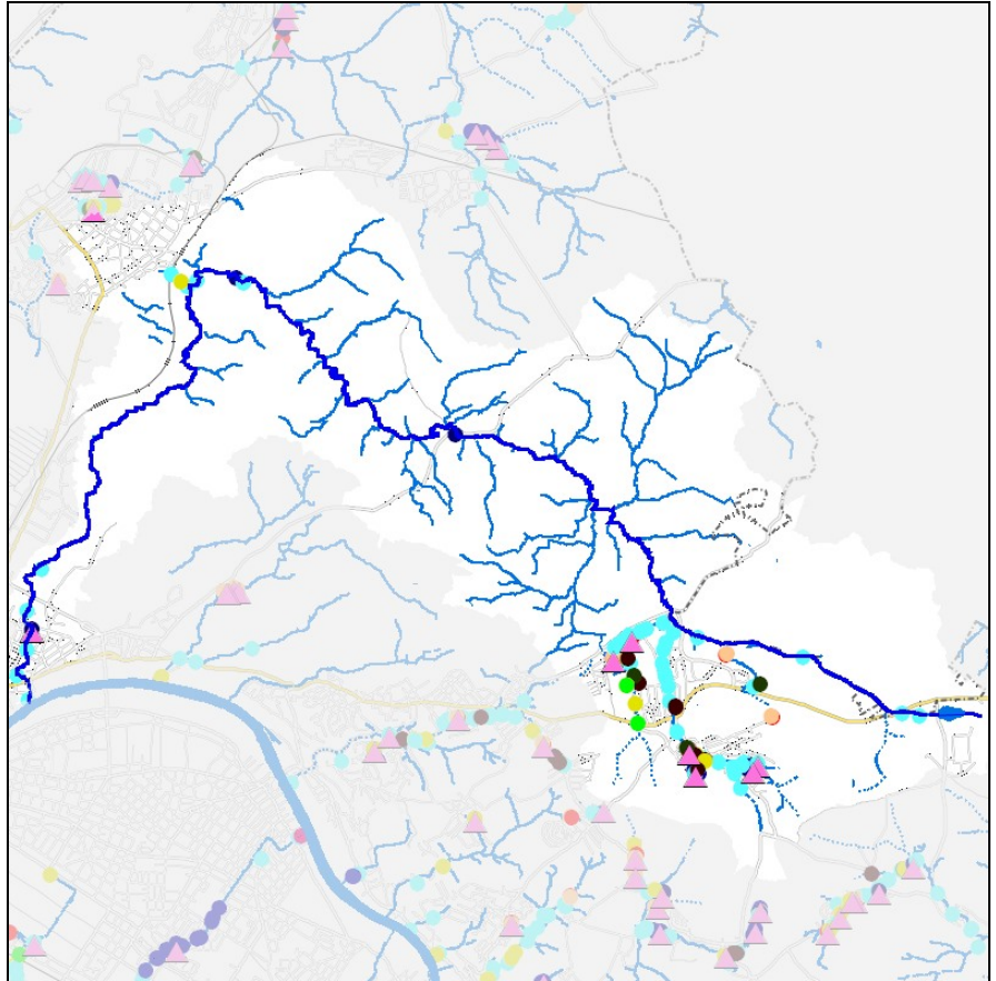
Abb. 31: Wasserwirtschaftliche Anlagen
