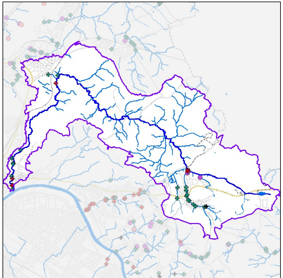
Abb. 35: Regenrückhaltebecken und wesentliche Einleitungen aus dem Kanalnetz
