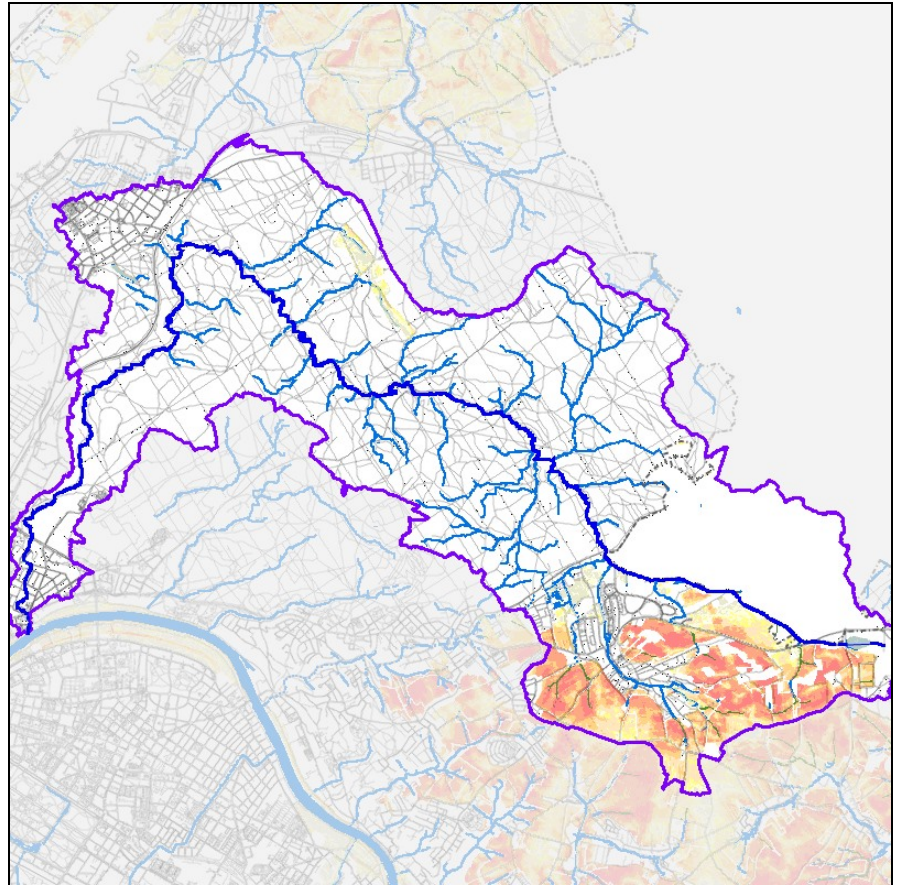
Abb. 38: Potentielle Erosion nach ABAG im Einzugsgebiet des Prießnitz
