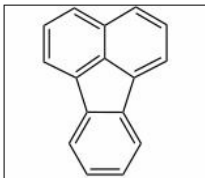
Abb. 13: Strukturformel Fluoranthen; 16.05.2018
