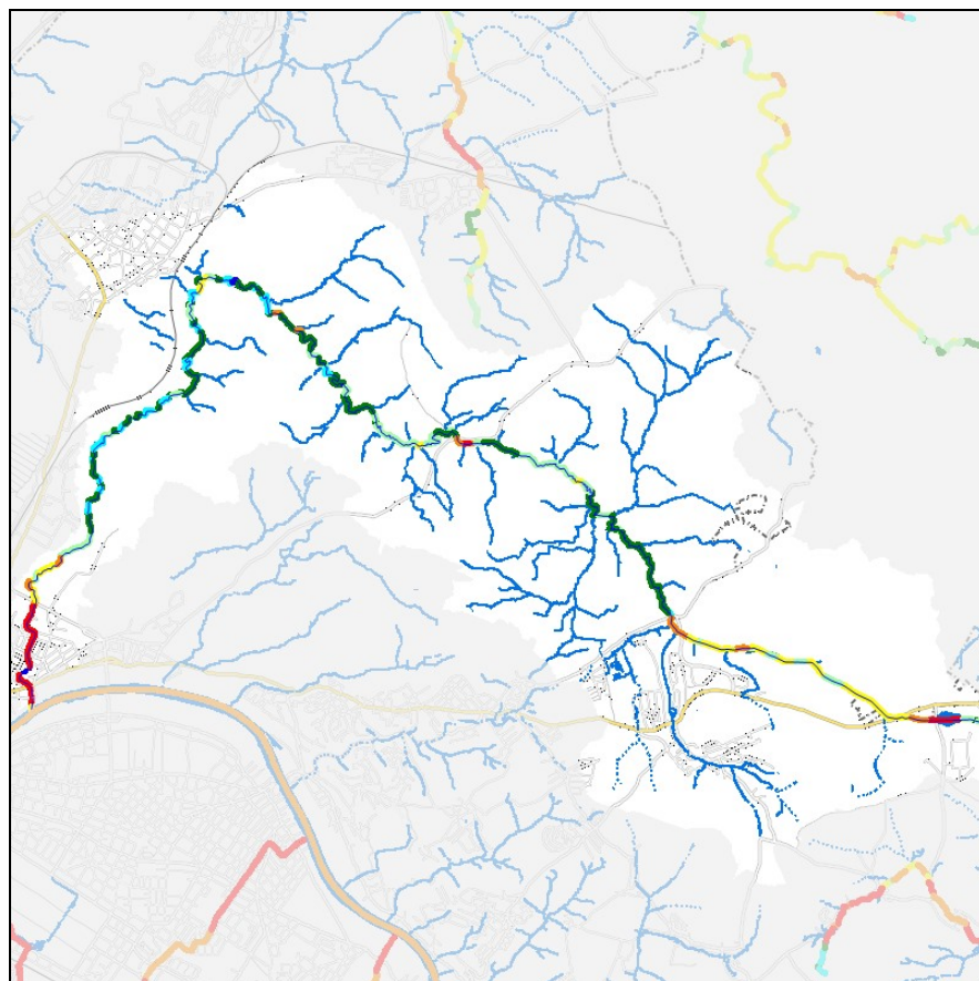
Abb. 12: Gewässerstrukturgüte LfULG, Stand 2016 Prießnitz
