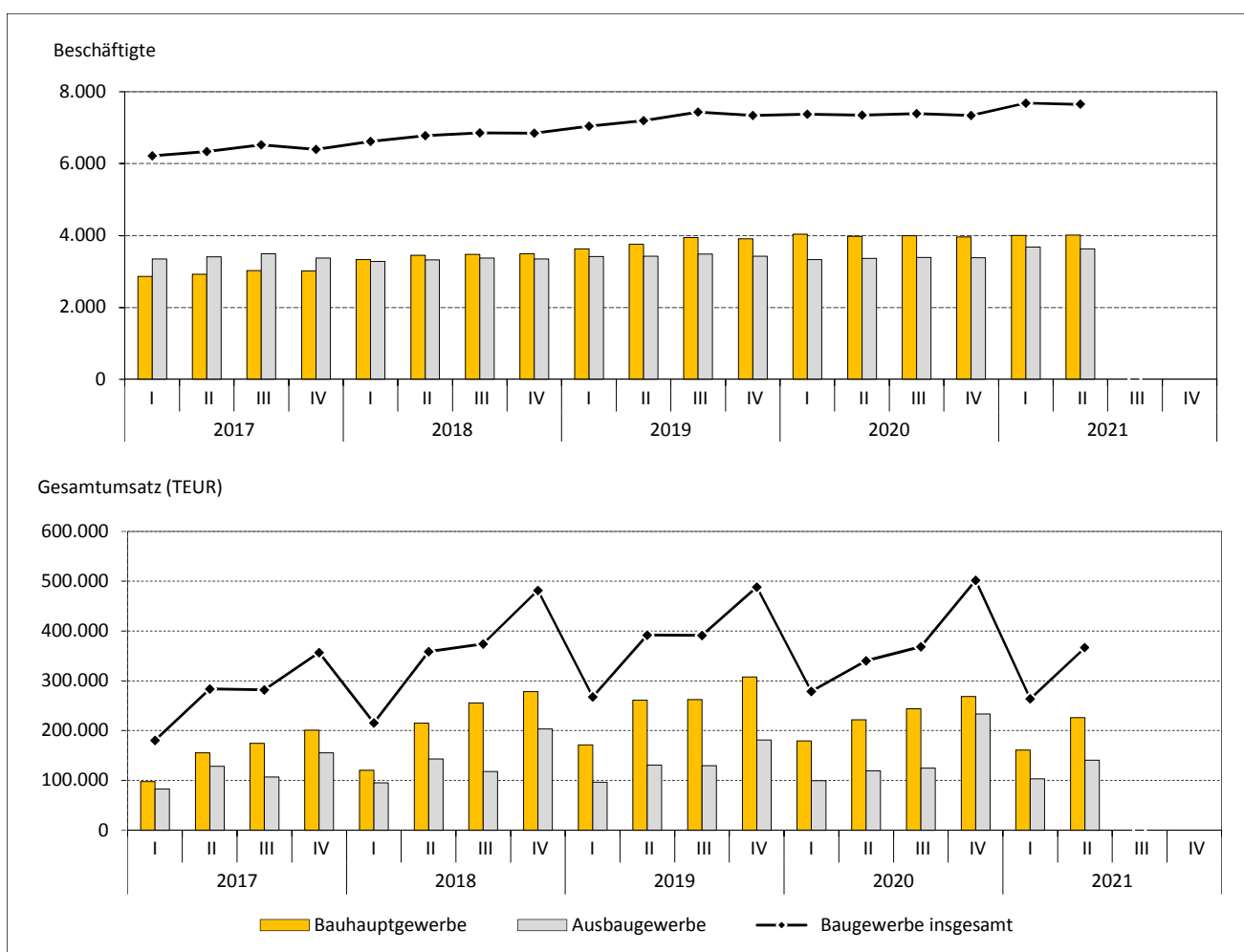
Abb. 1: Beschäftigte und Gesamtumsatz im Baugewerbe insgesamt 3)
