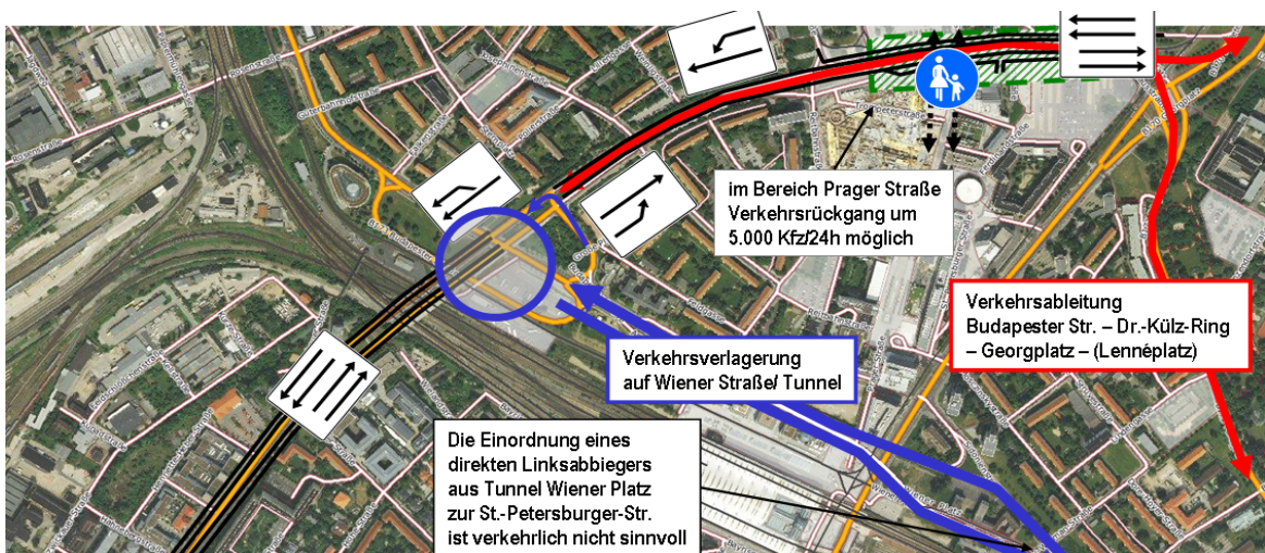
Grafik 5: Prinzipskizze Verkehrsableitung Dr.-Külz-Ring über Wiener Tunnel
