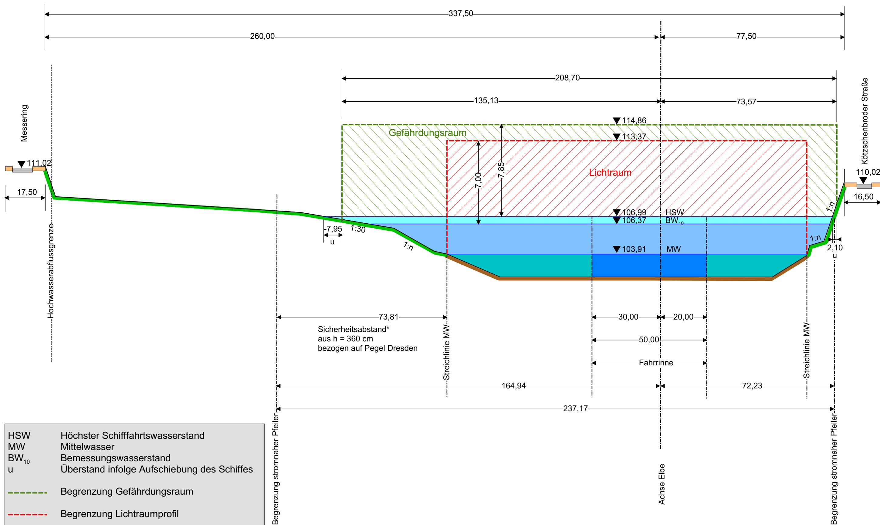
Prinzipskizze Querschnitt bei Wasserstraßenkilometer 58,725 (Bereich westlich Ballhaus Watzke)
