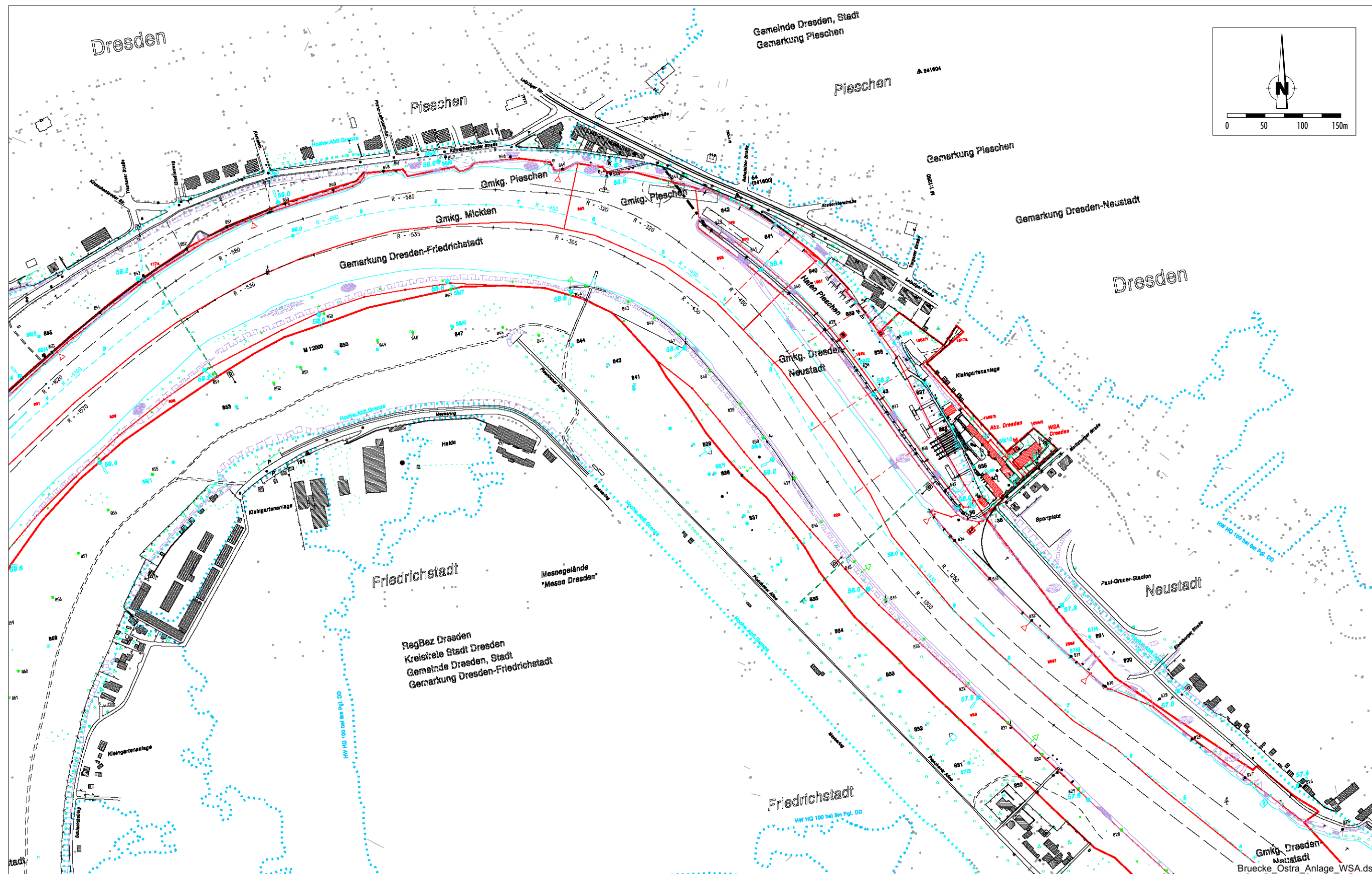
Auszug aus der Wasserstraßenkarte Elbe, Quelle: Wasser- und Schifffahrtsamt Dresden, Juli 2012
