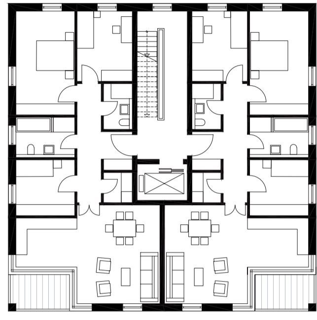
GRUNDRISS 2.OG HAUSTYP S 16,5X16,5m 2 X 4-ZIMMER WOHNUNGEN I M 1:200
