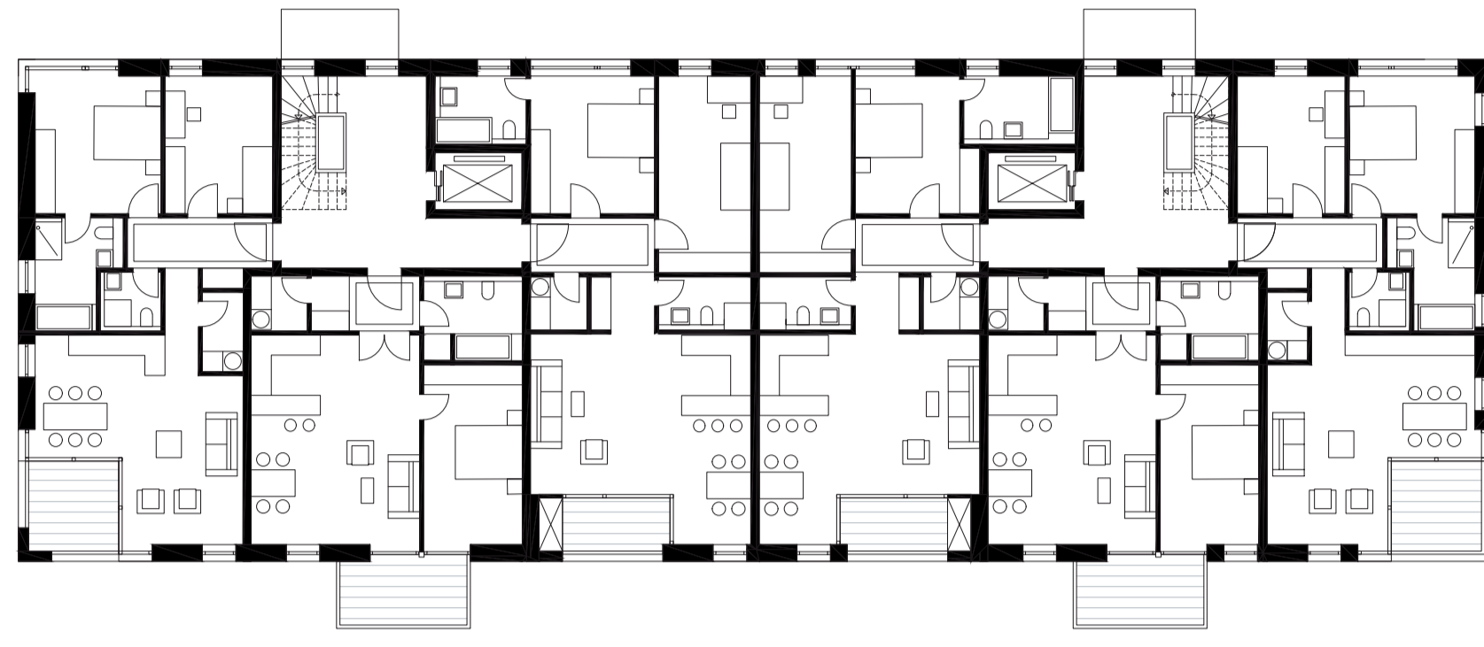
GRUNDRISS 2.OG HAUSTYP 2xM 22X15m 2 X 3-ZIMMER + 1 X 2-ZIMMER WOHNUNGEN I M 1:200
