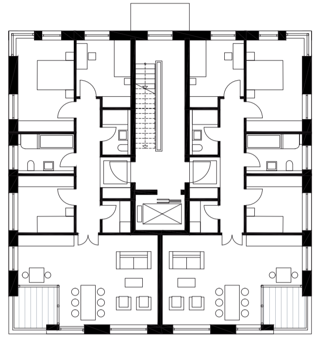
GRUNDRISS 2.OG HAUSTYP S 16,5X16,5m 2 X 4-ZIMMER WOHNUNGEN I M 1:200
