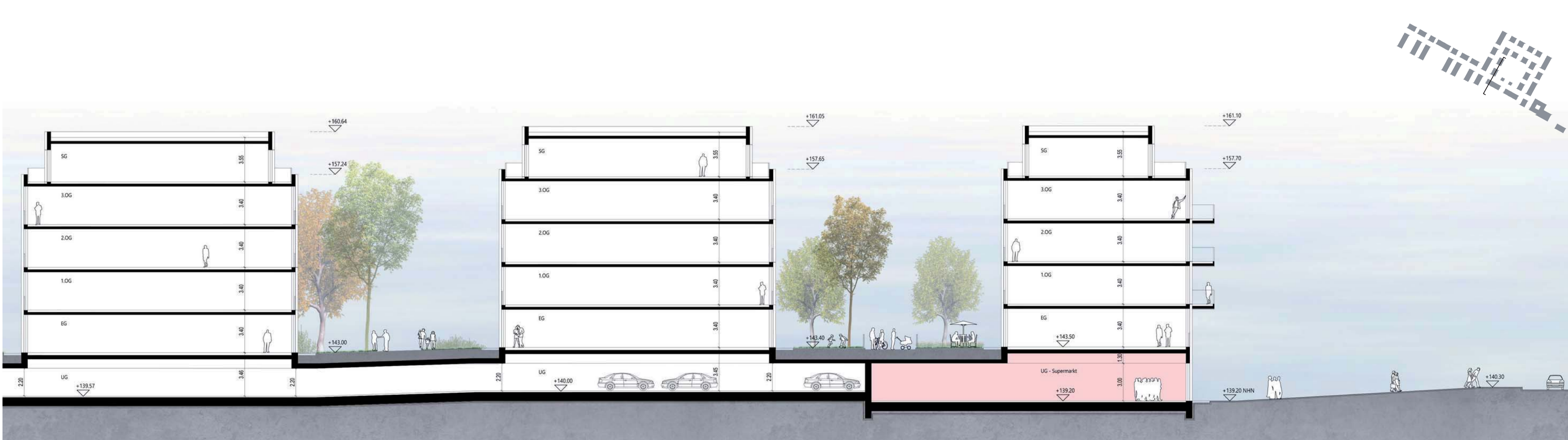
SCHNITT | M1:250
