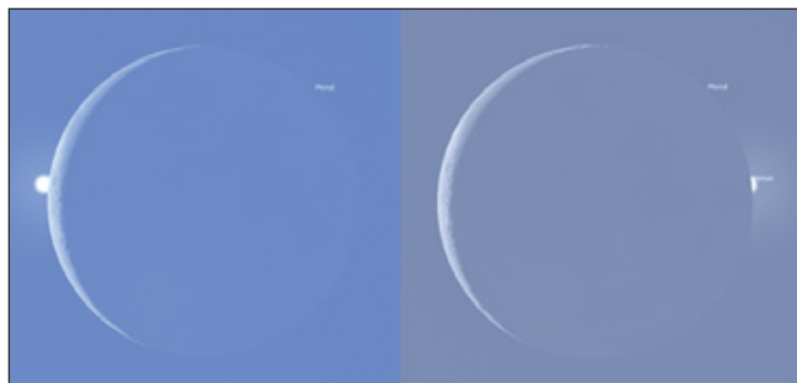
Bedeckung der Venus durch den Mond (Bild: Dr. Frank Bok, Stellarium)
