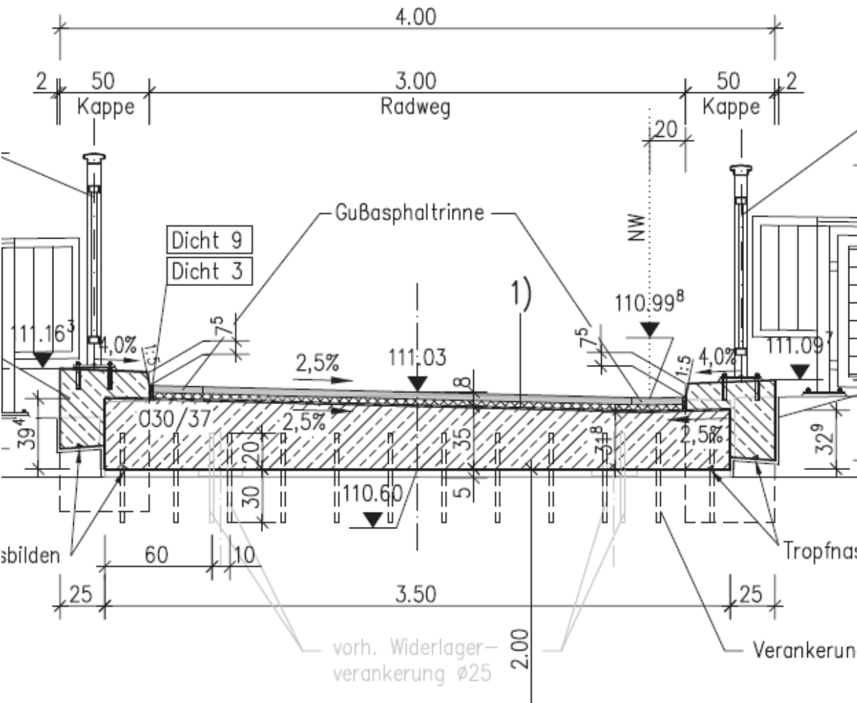
Querschnitt: Straßen- und Tiefbauamt
