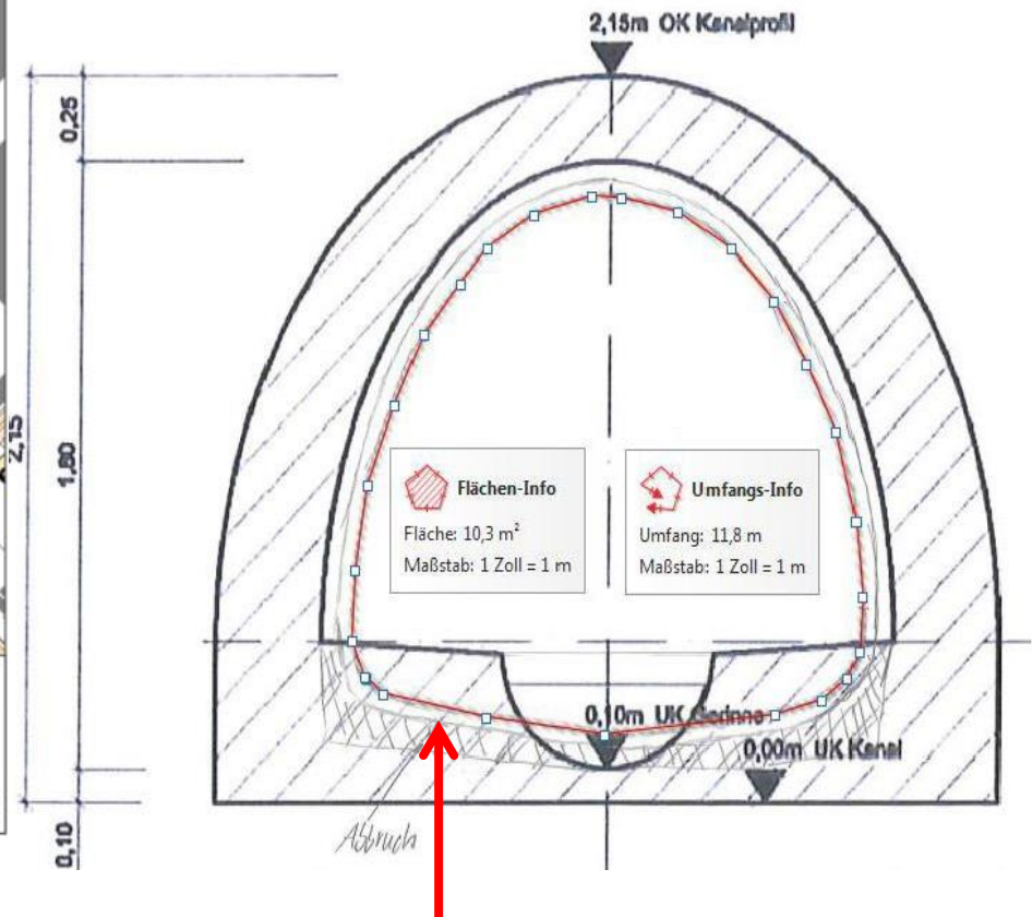
Inliner Ei-Profil
