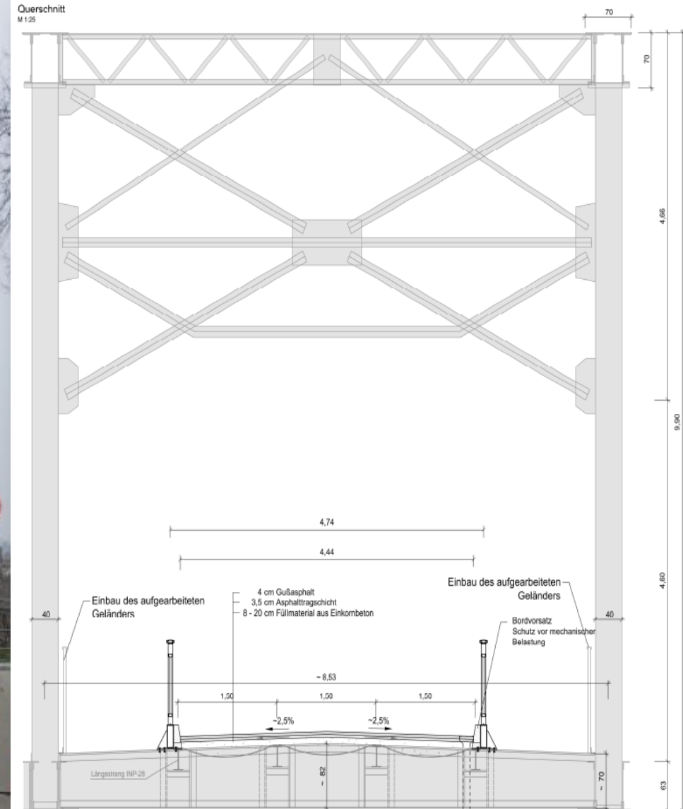
Querschnitt: Straßen- und Tiefbauamt
