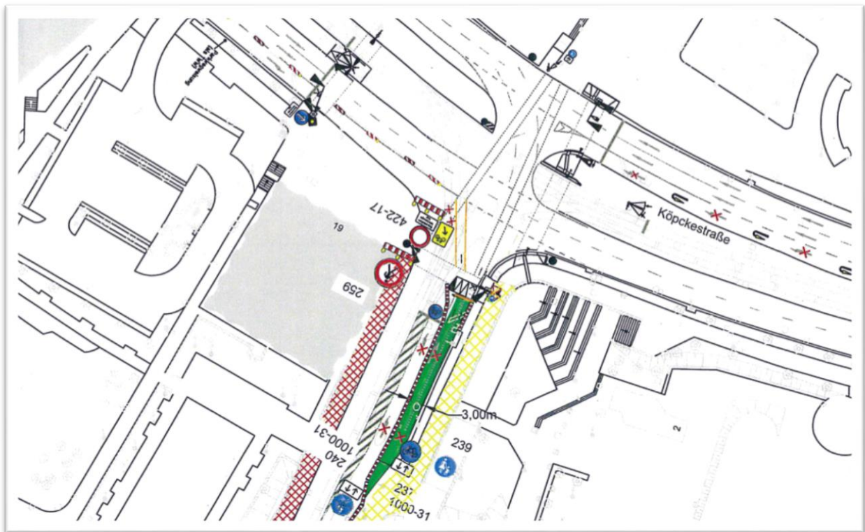
Abbildung 1 Verkehrsführung auf Neustädter Seite ab 23.08.
