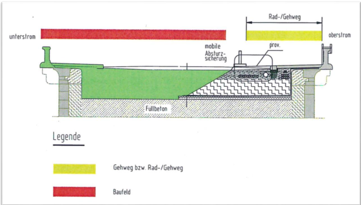
Abbildung 3 Abgrenzung Verkehrsfläche und Baubereich auf der Brücke ab 23.08.2019
