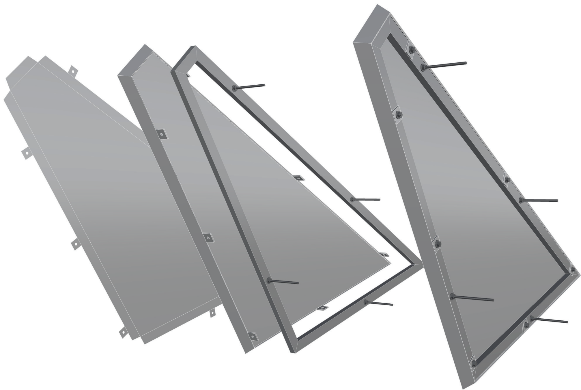
Konstruktionsaufbau am Beispiel eines Elements
